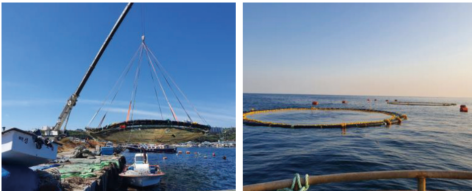
부상침하식 동합금망 해상가두리
